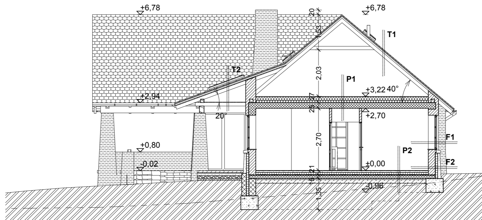
A1-A1 metszet
