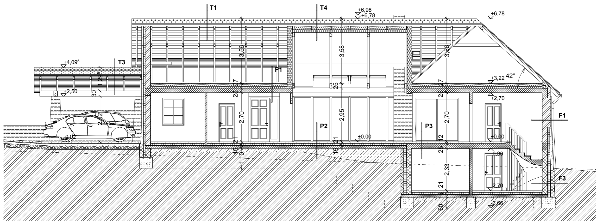
B1-B1 metszet
