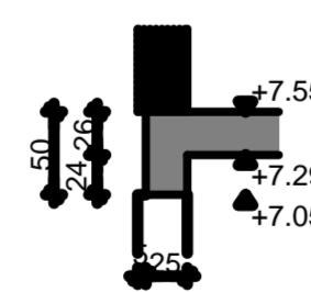
G-1, 25×50 cm Készül 29,60 fm
