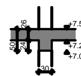
G-2, 30×50 cm Készül 20,30 fm
