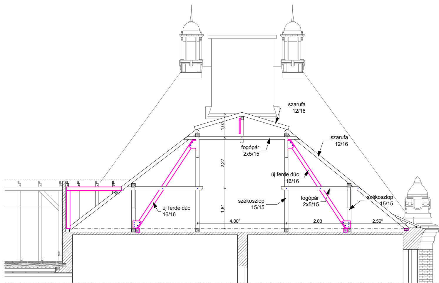
D1-C-C metszet
