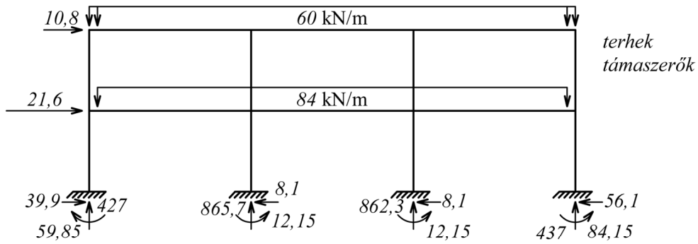
Függőleges és vízszintes terhek együttes hatása
